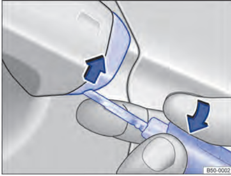
Fig. 56 Manilla de la puerta del conductor: levantar la caperuza.
