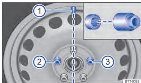
Fig. 218 Cambio de rueda: válvula del neumático ① y posición de montaje del tornillo de la rueda antirrobo ② o ③.
