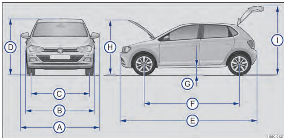
Fig. 227 Dimensiones.
