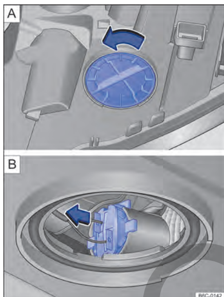
Fig. 182 Farol delantero, por debajo: cubierta del indicador de dirección.
