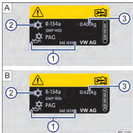
Fig. 226 A : Información del aire acondicionado - motor 1.0L. B : información del aire acondicionado - motor 1.0L TSI, motor 1.4L TSI y motor 1.6L.
