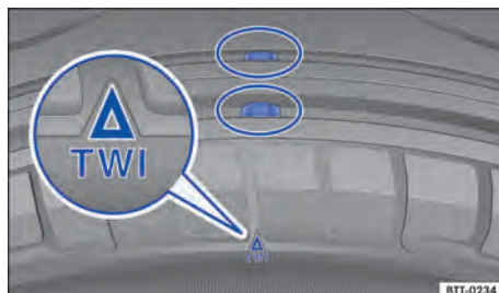
Fig. 212 Perfil del neumático: indicadores de desgaste.
