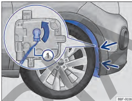
Fig. 186 En la caja de la rueda delantera: acceso a la bombilla del faro de neblina.
