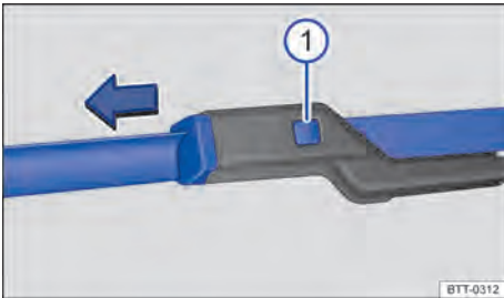
Fig. 183 Sustituir las escobillas de los limpiaparabrisas.
