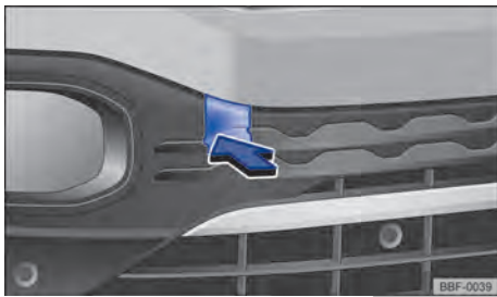
Fig. 198 En el parachoques delantero a la derecha: suelte y desmonte la cubierta.
