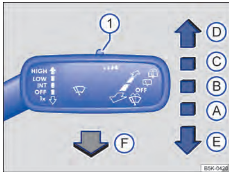
Fig. 76 A la derecha de la columna de dirección: comandar los limpiavidrios.
