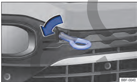
Fig. 199 En el parachoques delantero a la derecha: enrosque la argolla de remolque.
