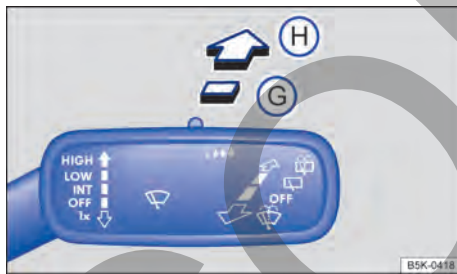
Fig. 77 A la derecha de la columna de dirección: comandar el lavavidrios.
