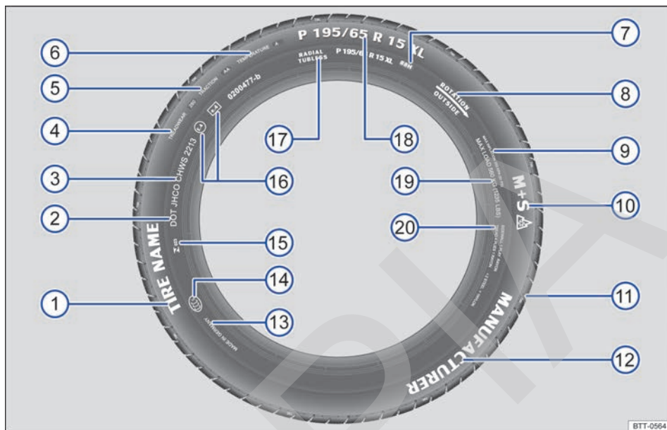
Fig. 144 Inscripción en los neumáticos internacional (ejemplo).
