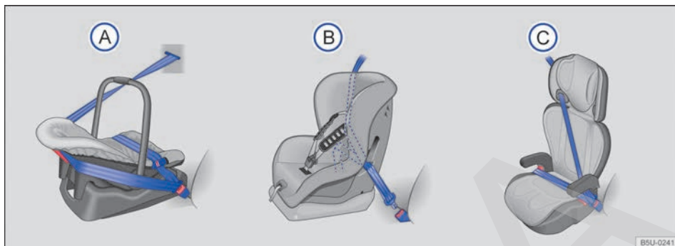
Fig. 57 Las ilustraciones (A), (B) y (C) muestran la fijación del sistema de retención infantil sólo con el cinturón de seguridad del vehículo.
