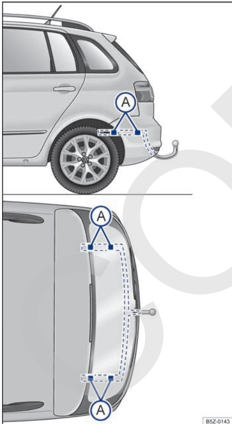
Fig. 81 Puntos de fijación para el montaje posterior de un enganche para remolque.
