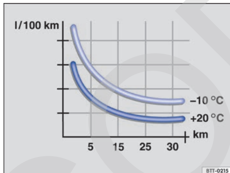
Fig. 112 Consumo de combustible en l/100 km en 2 temperaturas ambiente diferentes.
