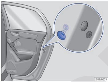
Fig. 59 En la puerta trasera (lado derecho): ubicación del seguro para niños.
