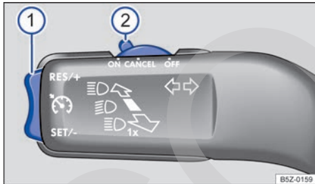
Fig. 120 A la izquierda en la columna de la dirección: palanca de manejo del GRA.
