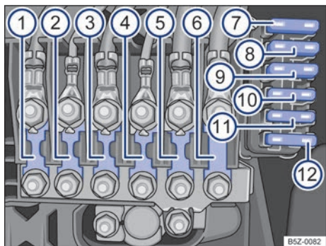
Fig. 171 Caja de fusibles.
