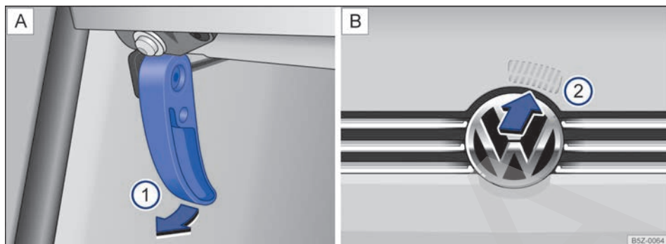
Fig. 127 A: palanca de desbloqueo en la zona reposapiés del lado del conductor (1). B: palanca de desbloqueo en la parte interior de la tapa del compartimento del motor (2).
