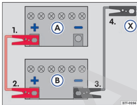
Fig. 184 Esquema para la conexión de los cables auxiliares de arranque: batería del vehículo descargada (A) y batería del vehículo que provee la corriente (B) .
