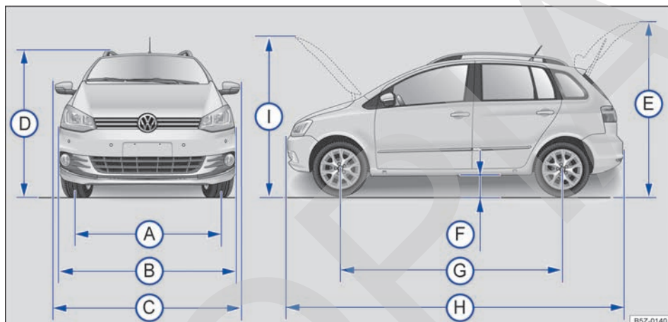
Fig. 19 Dimensiones.
