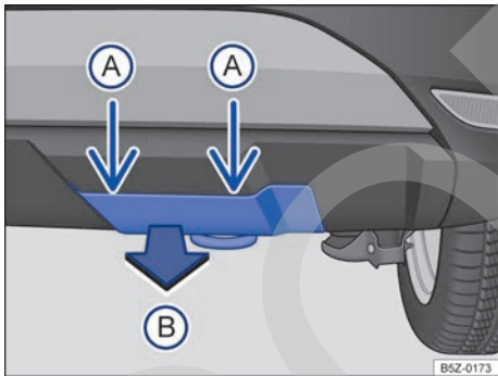
Fig. 190 En el paragolpes trasero a la derecha: argolla para remolque trasera - paragolpes con cubierta desmontable.
