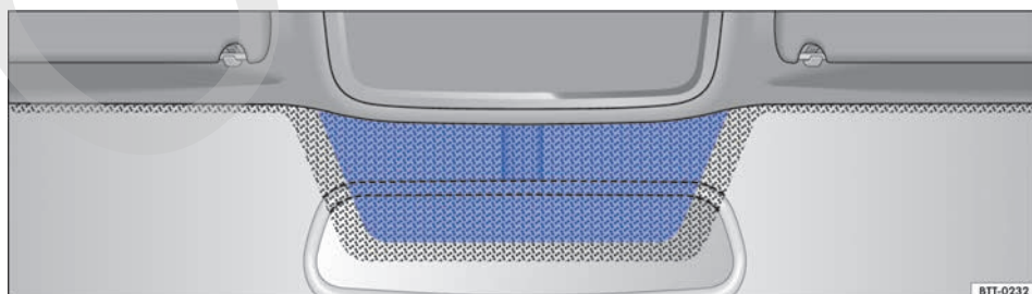
Fig. 64 Parabrisas con infrarrojo y revestimiento metálico con ventana de comunicación (superficie azul).
