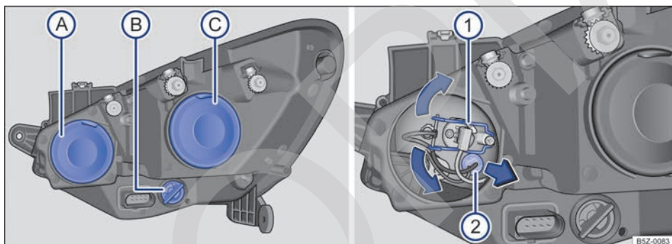
Fig. 172 En el compartimento del motor: vista trasera del farol delantero derecho con cubierta de goma (izquierda): A farol alto y luz de posición, B indicadores de dirección y C farol bajo. Vista trasera del farol delantero derecho sin cubierta de goma (derecha): 1 farol alto, 2 luz de posición.
