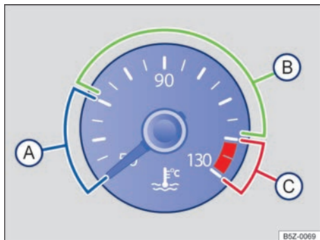
Fig. 131 Indicador de temperatura del líquido de refrigeración del motor en el panel de instrumentos: (A) zona fría; (B) zona normal; (C) zona de alerta.
