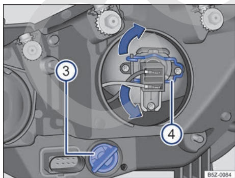
Fig. 173 En el compartimento del motor: vista trasera del farol delantero derecho sin cubierta de goma: 3 indicadores de dirección y 4 farol bajo.
