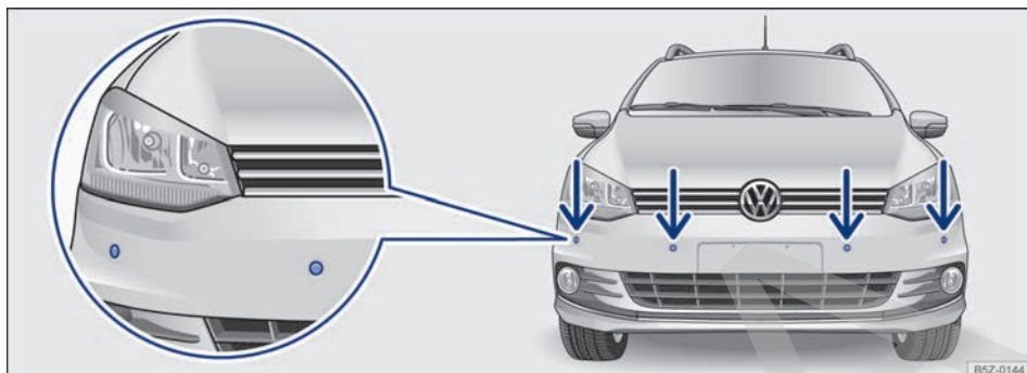
Fig. 115 Sensores de ultrasonido del control de distancia de aparcamiento en el parachoques delantero.
