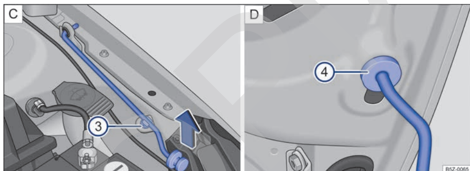
Fig. 128 C: varilla de sujeción de la tapa del compartimento del motor (3). D: tapa del compartimento del motor protegida con la varilla de sujeción de la tapa (4).
