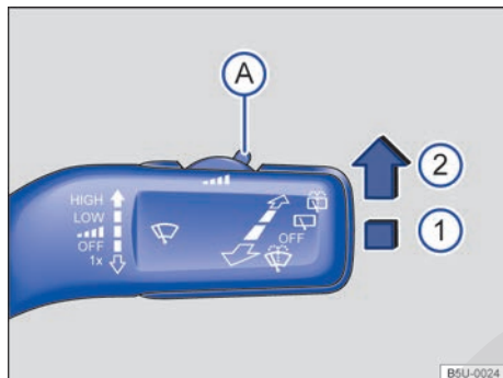
Fig. 66 Al lado del volante: palanca de los limpiavidrios: regular la sensibilidad del sensor de lluvia A .
