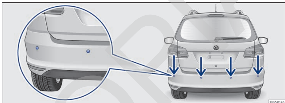
Fig. 116 Sensores de ultrasonido del control de distancia de aparcamiento en el parachoques trasero.
