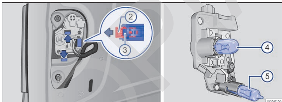
Fig. 180 En la tapa del maletero: soporte de las lámparas y lámparas de la linterna trasera izquierda - para vehículos con linterna de neblina.
