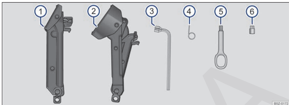
Fig. 159 Representación esquemática: componentes de las herramientas de a bordo.
