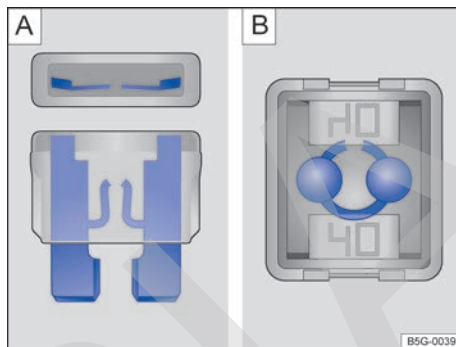
Fig. 239 Fusible fundido: A Fusible enchufable plano. B Fusible tipo bloque.
