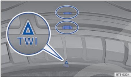
Fig. 264 Perfil del neumático: indicadores de desgaste.
