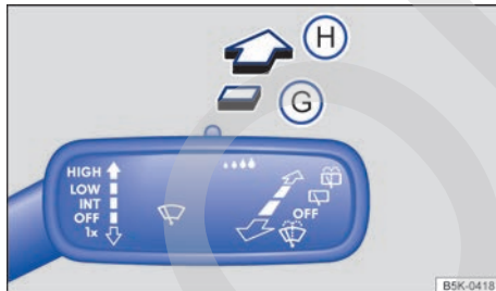
Fig. 112 En el lado derecho de la columna de dirección: manejo del limpialuneta (Variant).
