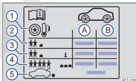
Fig. 262 Símbolos en el adhesivo de la presión de los neumáticos.
